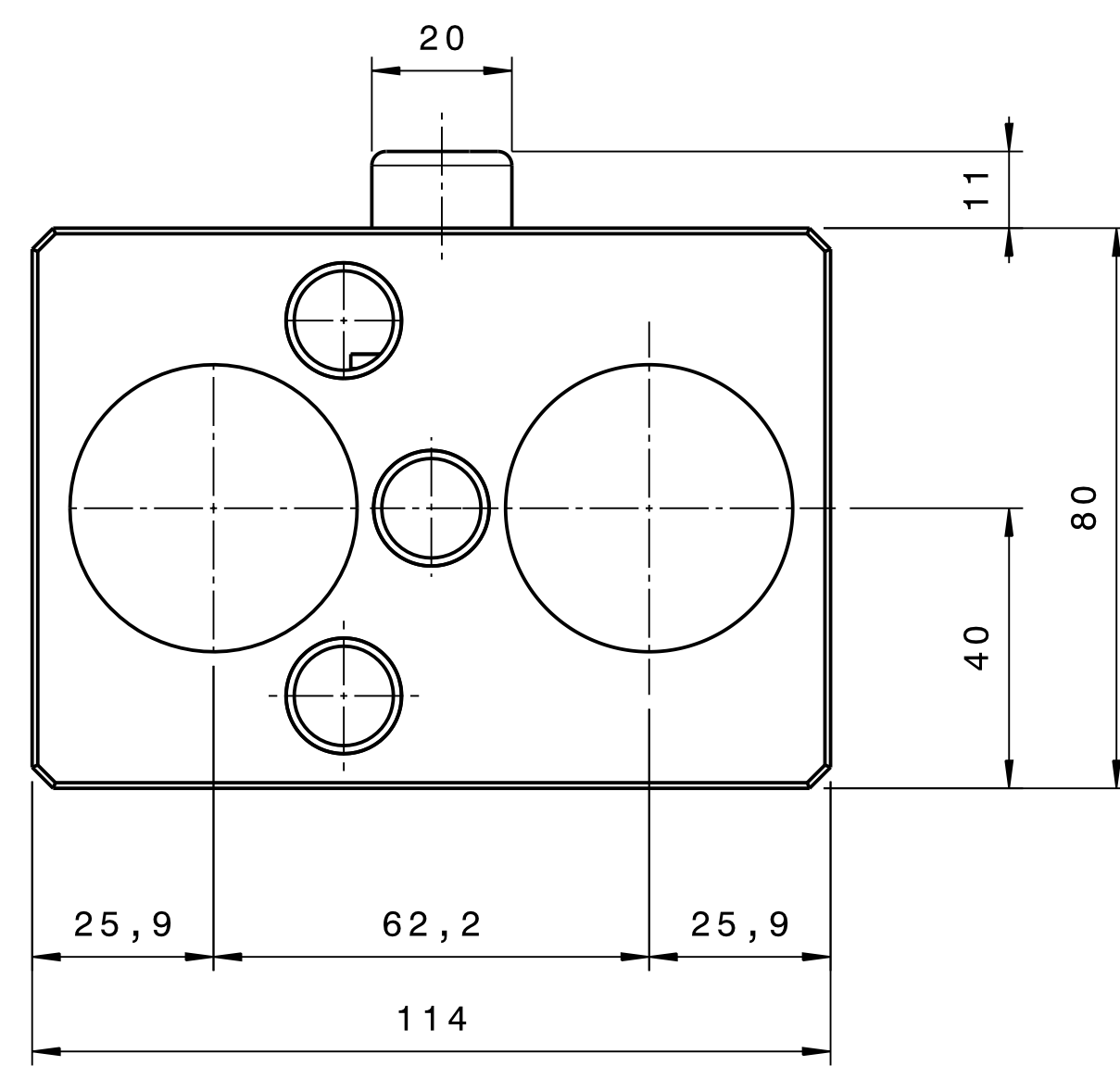
VORDERANSICHT
