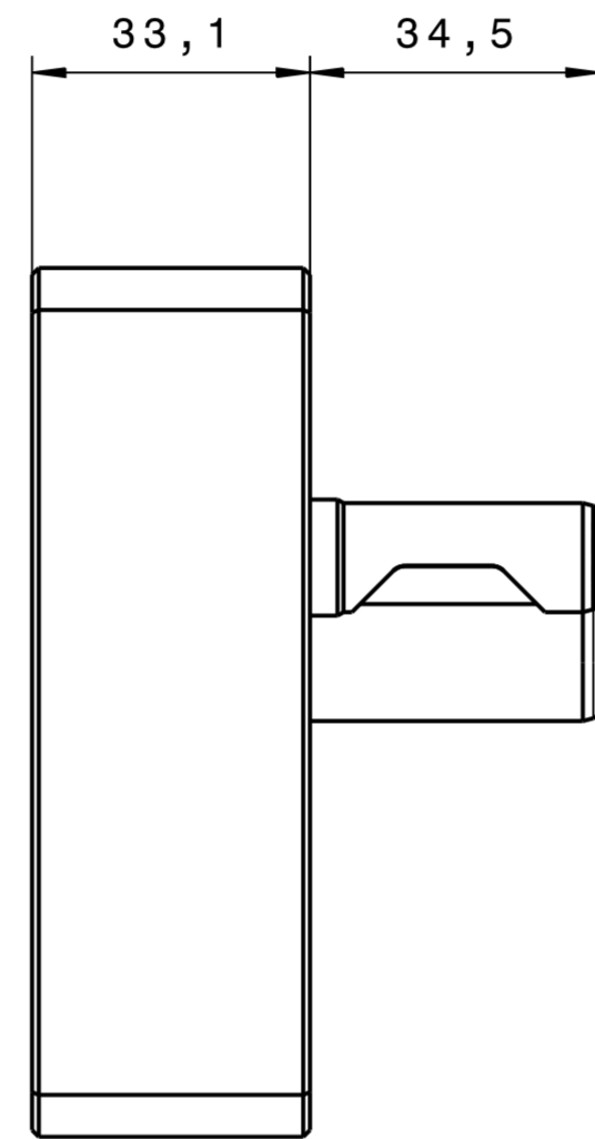
SEITENANSICHT LINKS
