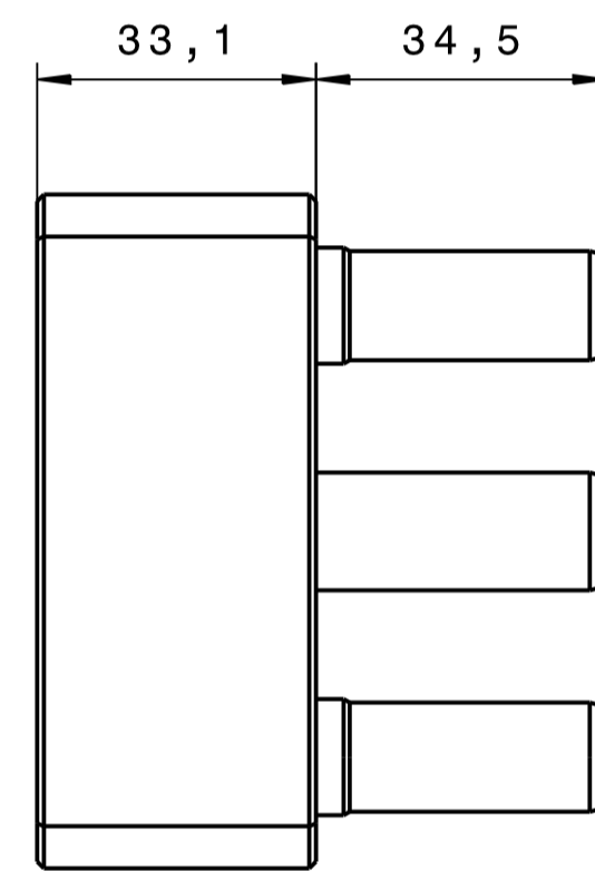
SEITENANSICHT LINKS
