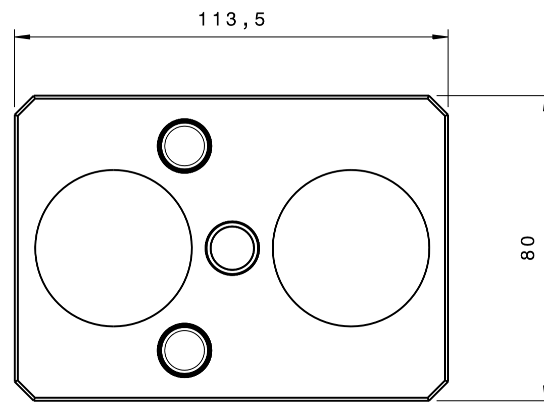
VORDERANSICHT
