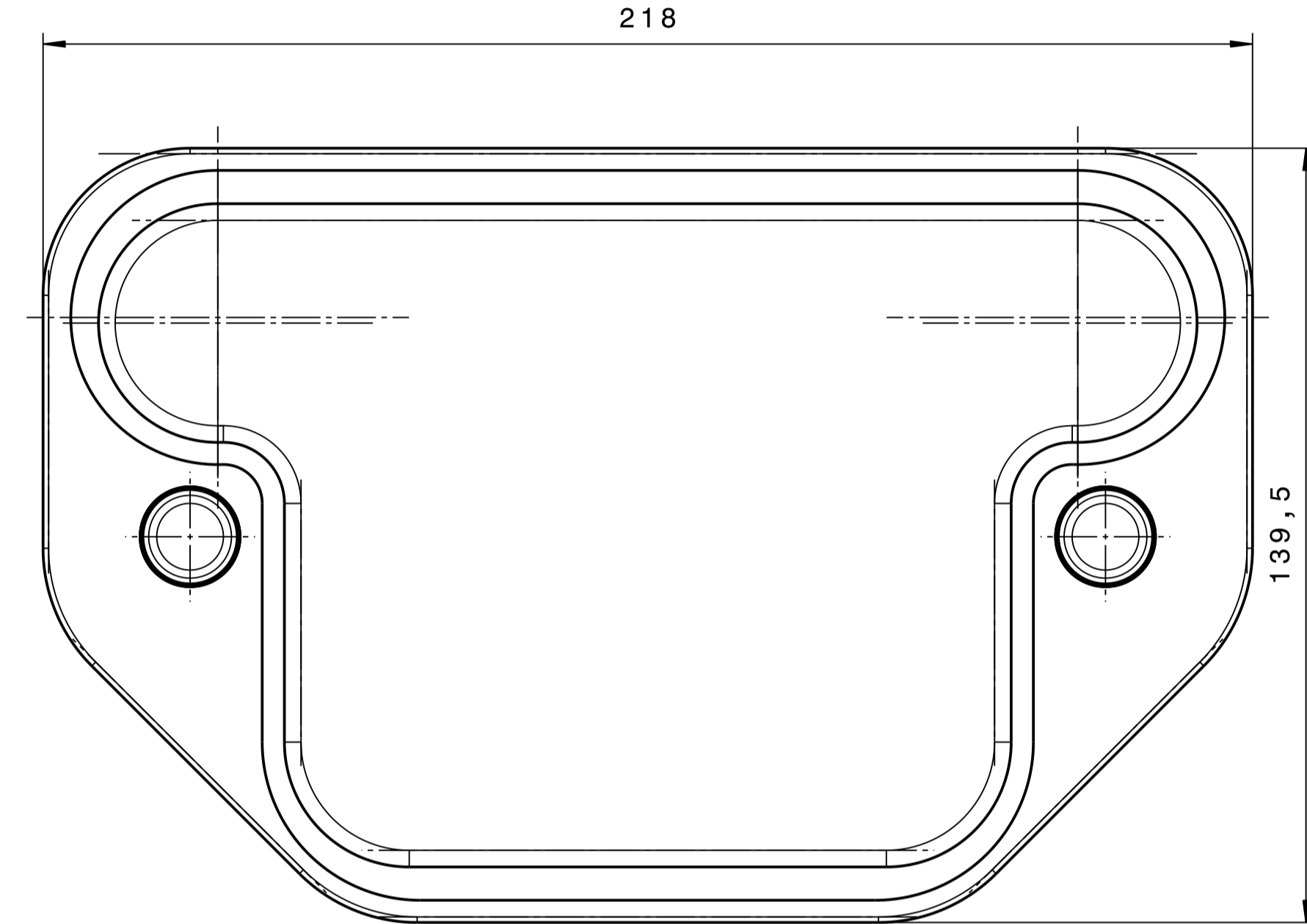
VORDERANSICHT
