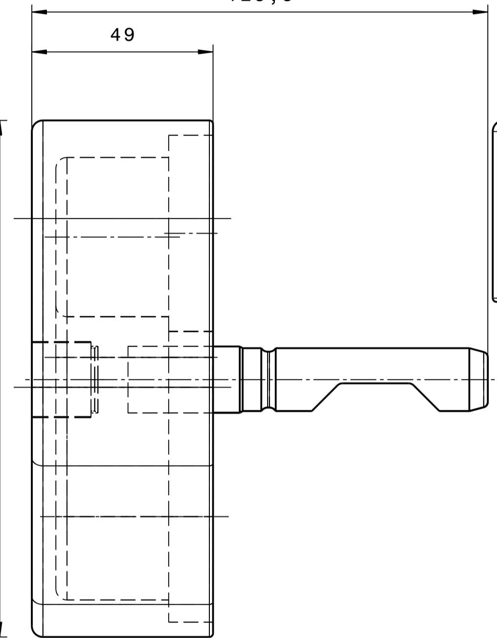
SEITENANSICHT LINKS
