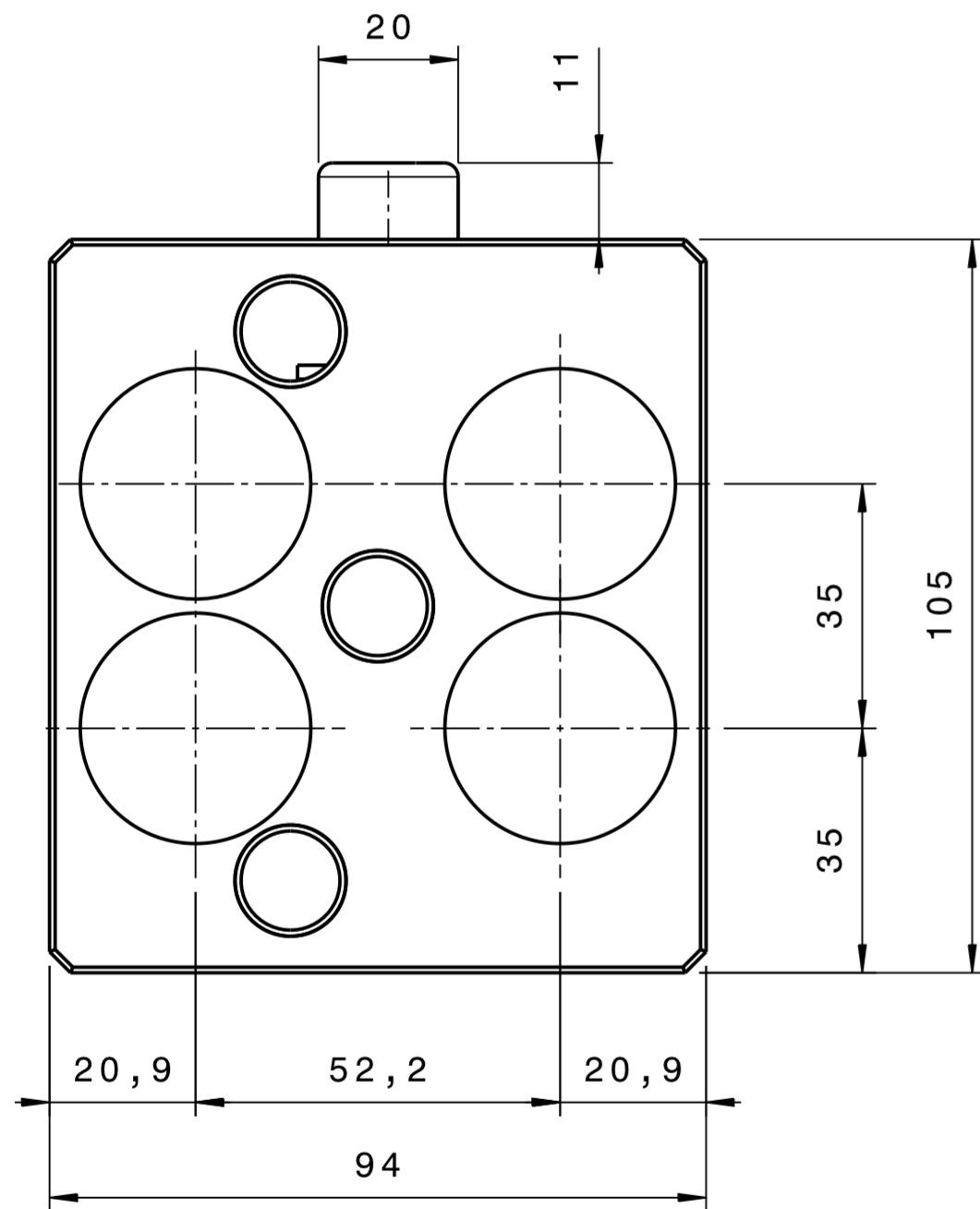
VORDERANSICHT
