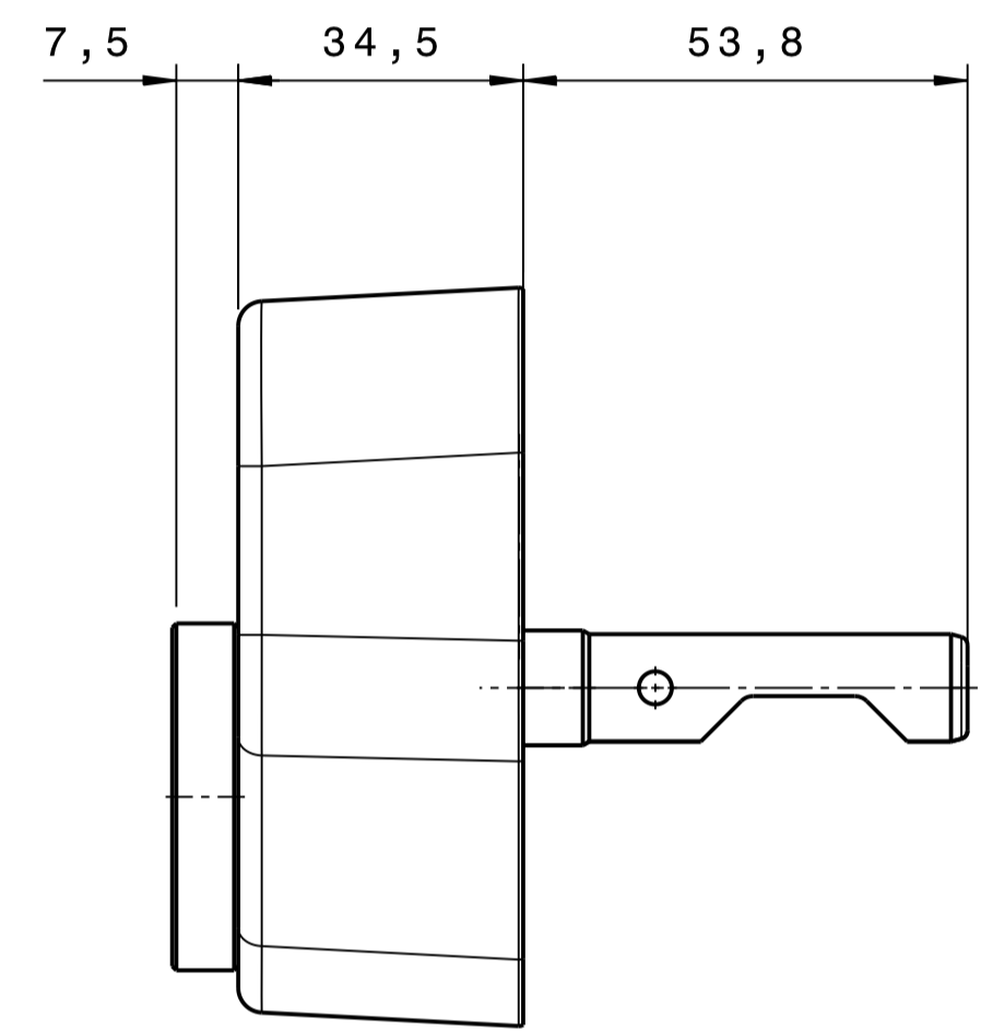
SEITENANSICHT LINKS
