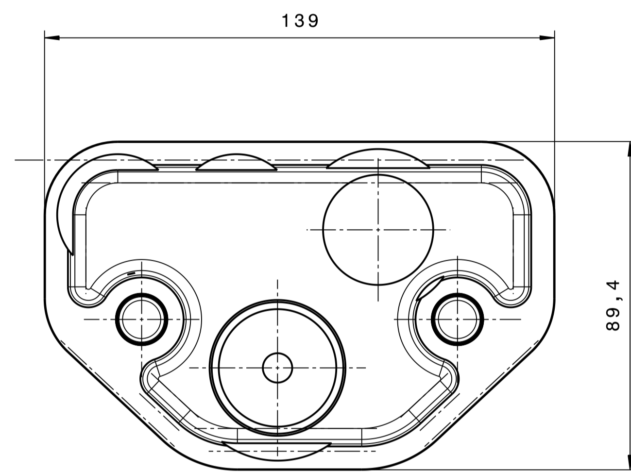
VORDERANSICHT
