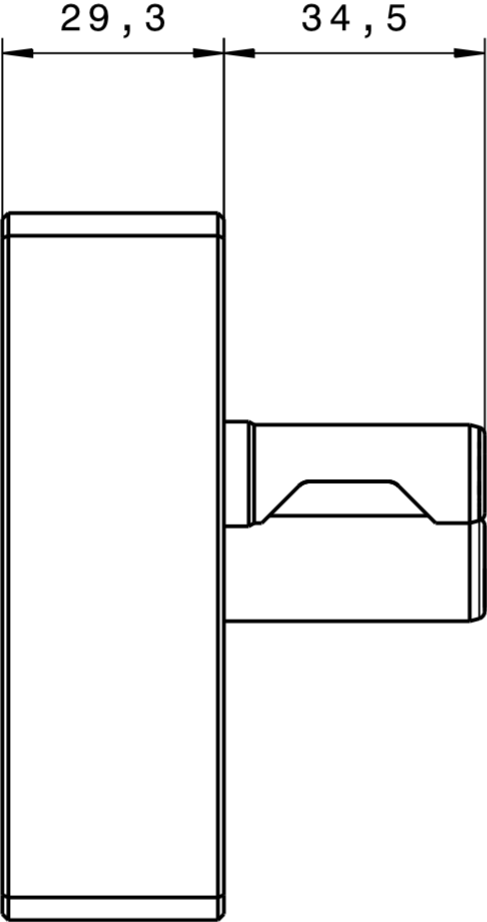
SEITENANSICHT LINKS
