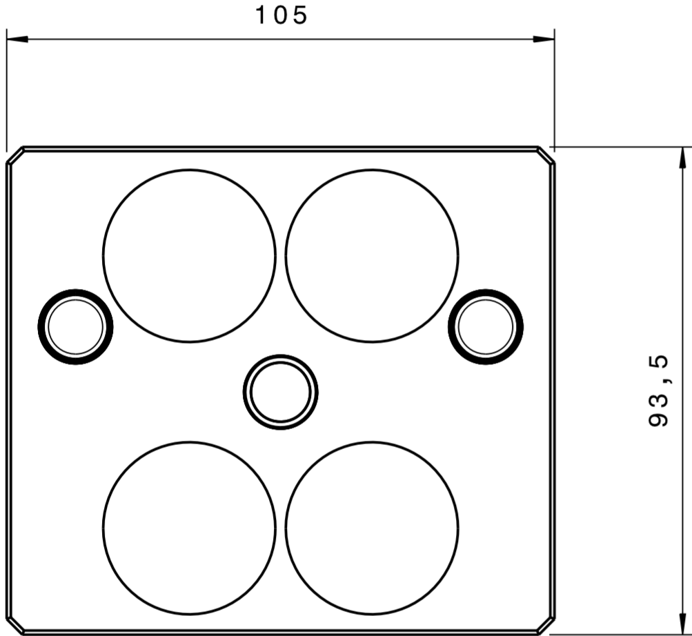
VORDERANSICHT
