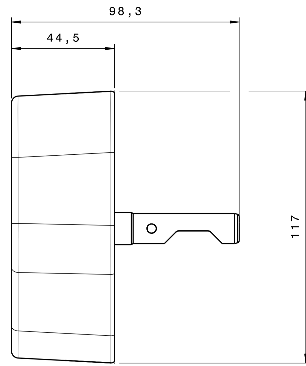
SEITENANSICHT LINKS
